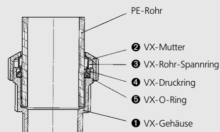
Schnittmodell einer VX-Klemmverbindung »Gerade Form« Mit Mutter und Außengewinde
